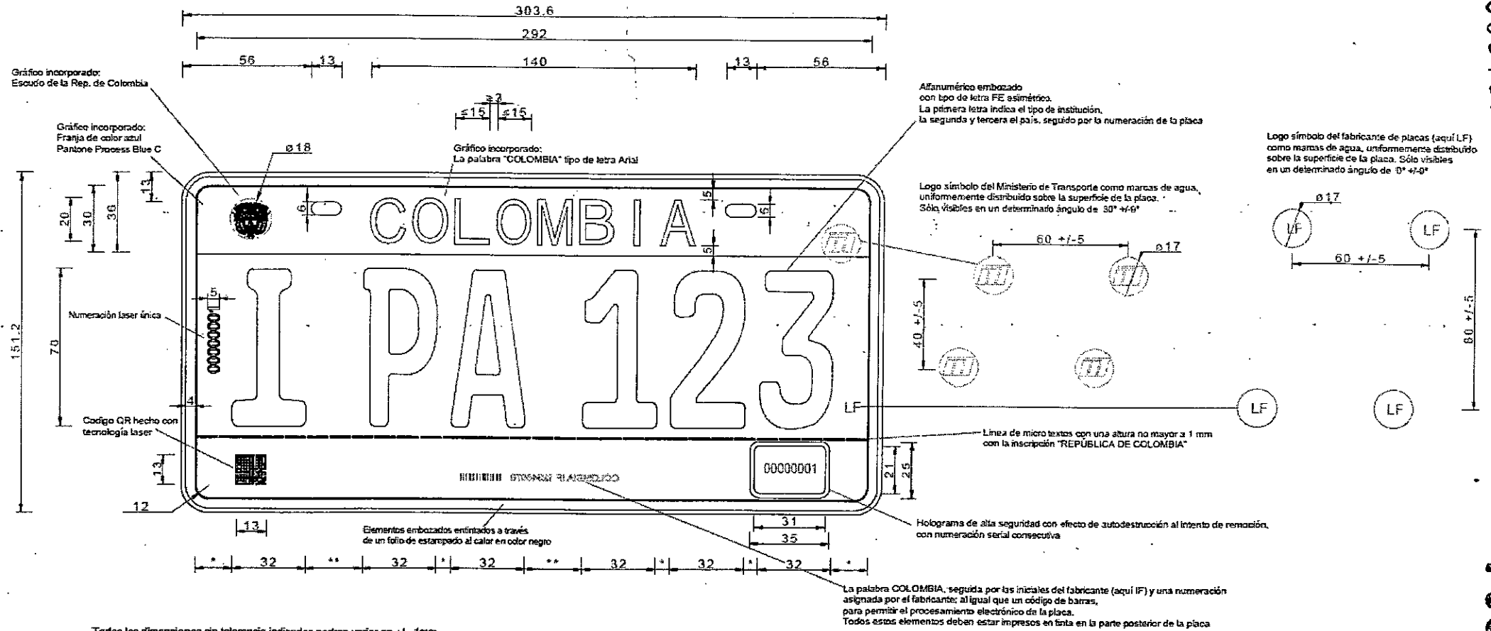
FIGURA No. 1 DISEÑO TECNICO DE LA PLACA PARA VEHÍCULO AUTOMOTOR
